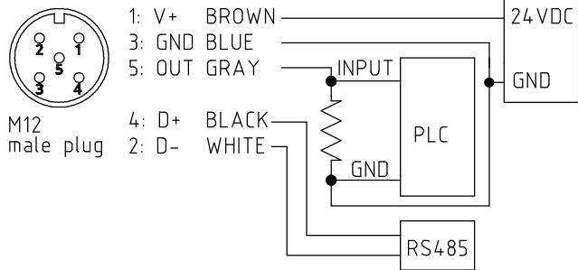
PNP 警報，RS485 輸出
